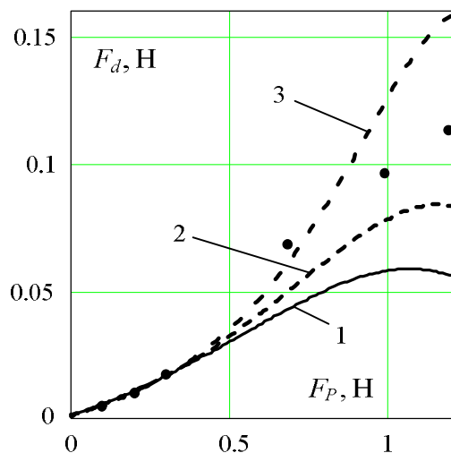
Рис. 5. Залежність вхідного сигналу перетворювача F_d від сили його притискування F_p до поверхні зони реєстрації пульсового сигналу (“поверхнєве” розташування променевої артерії)
