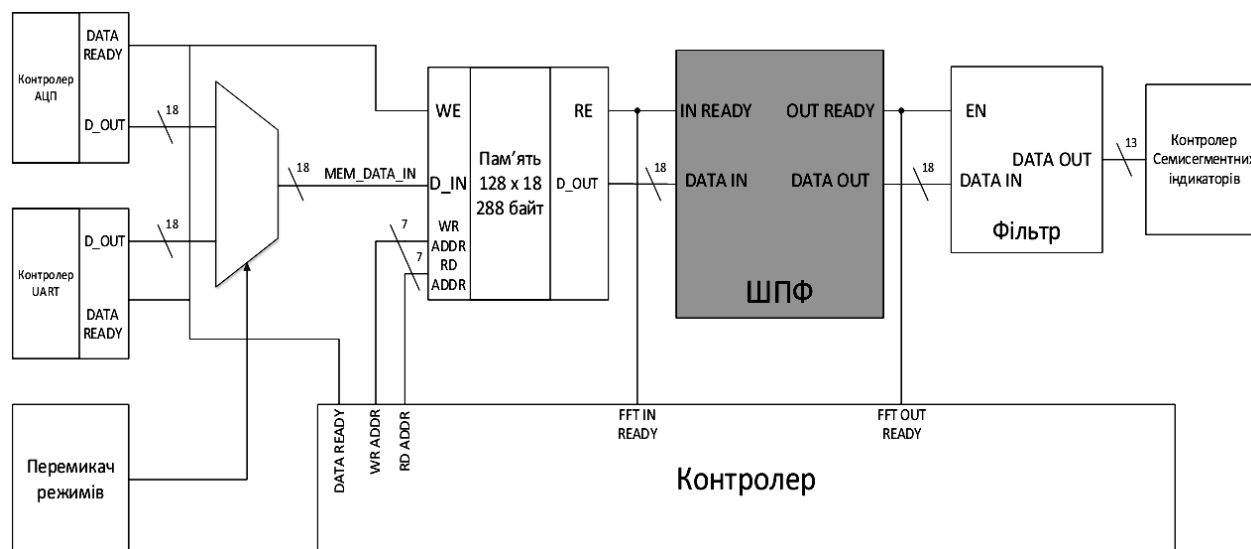
Рис. 5. Функціональна схема інструментальних засобів для дослідження характеристик процесорів 64-точкового ШПФ, генерованих системою "Хамелеон"
