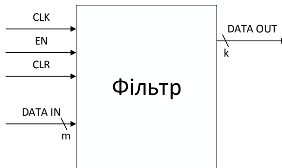
Рис. 7. Інтерфейс фільтра:
