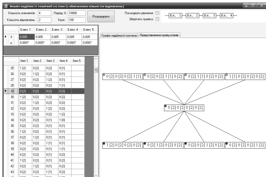
Рис. 7. Візуалізація фрагмента графу станів та переходів
