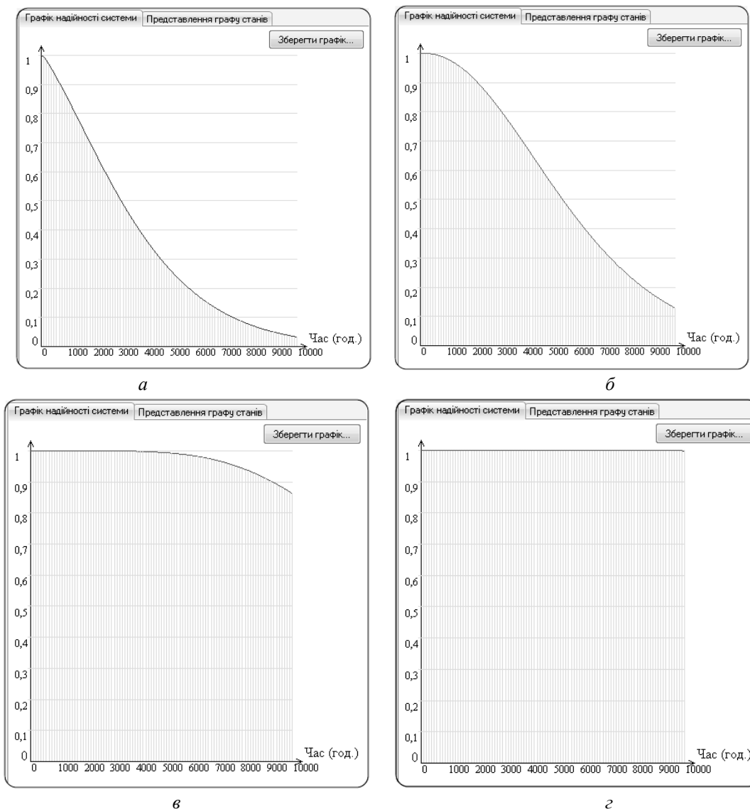
Рис. 5. Часові залежності ймовірності безвідмовної роботи системи для різних варіантів її побудови та відновлення: а – 4 елементи з 1-м відновленням; б – 3 елементи з 2-ма відновленнями; в – 2 елементи з 6-ма відновленнями; г – 2 елементи з 10-ма відновленнями
