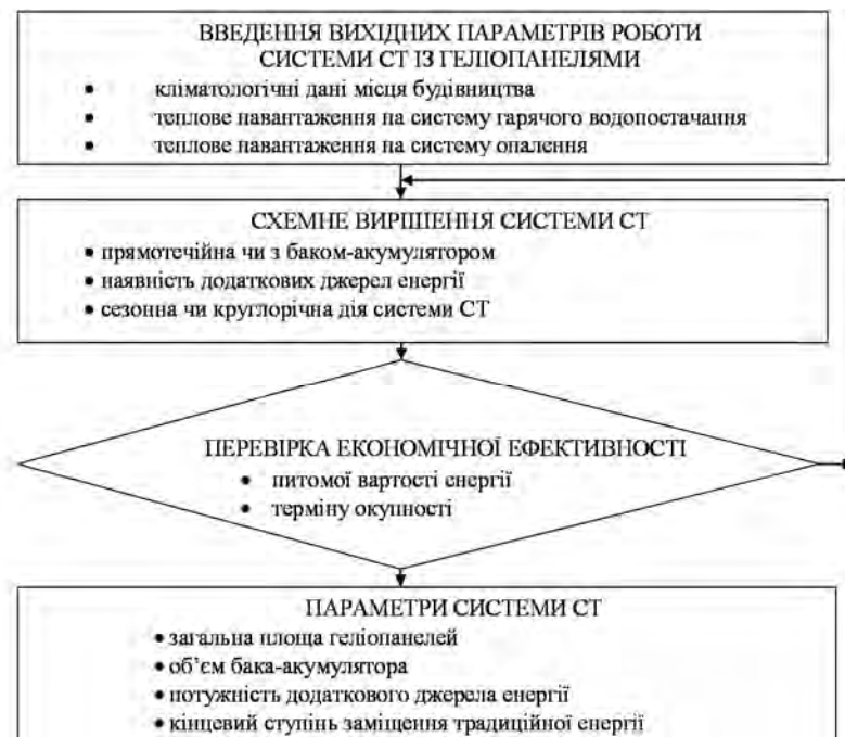
Алгоритм розрахунку параметрів системи сонячного тепlopостачання
