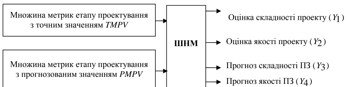
Рис. 2. Концепція НМОП
