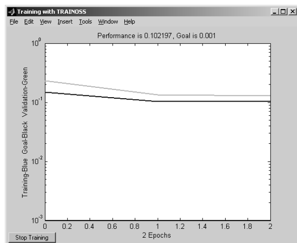
Рис. 4. Навчання і тестування нейромережі за методом OSS
