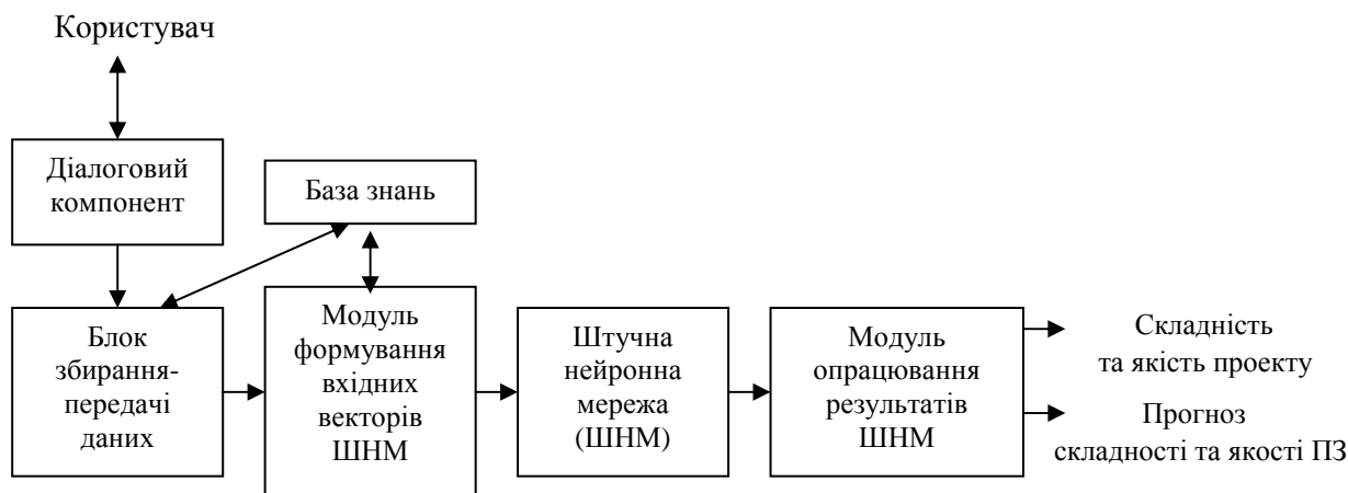
Рис. 5. Структурна схема ІСОП
